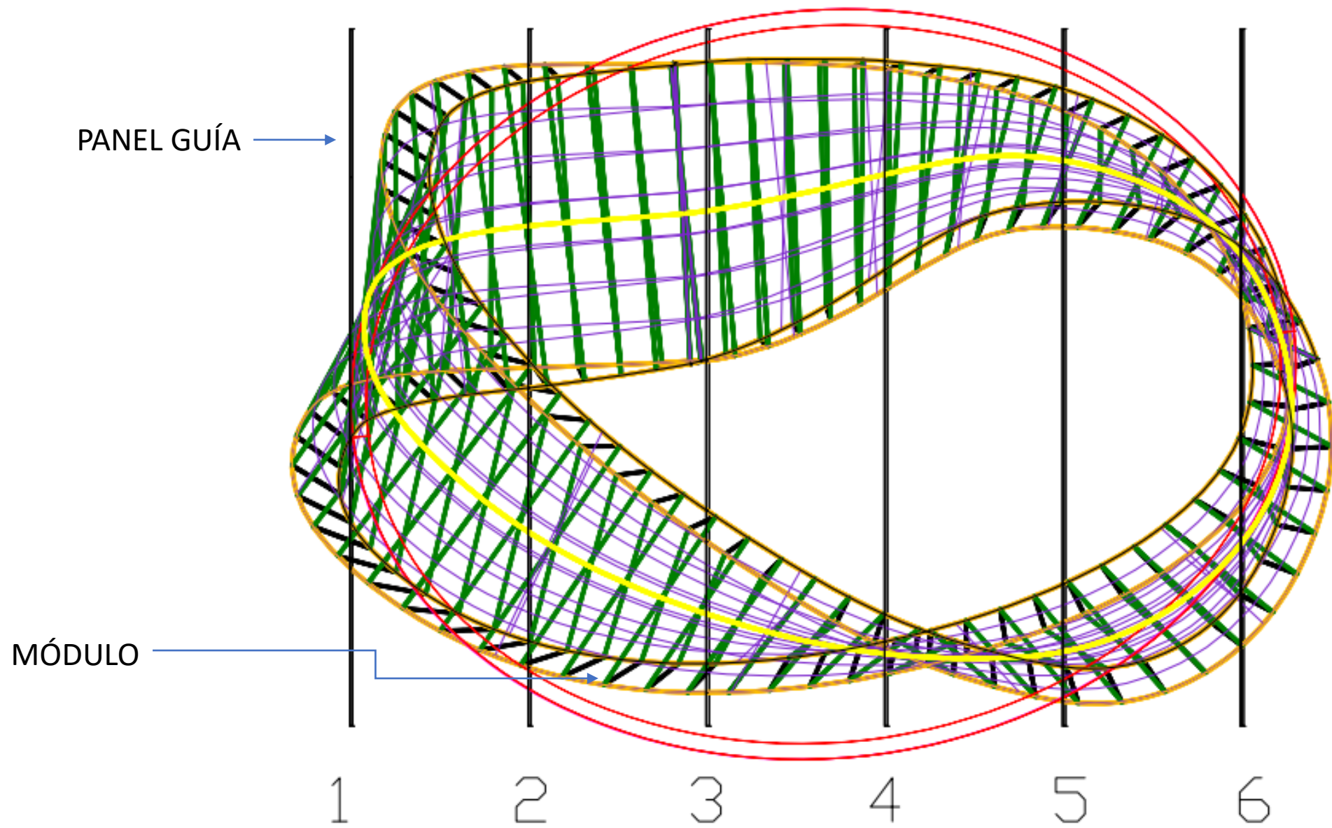
ESTRUCTURA EN PLANTA
